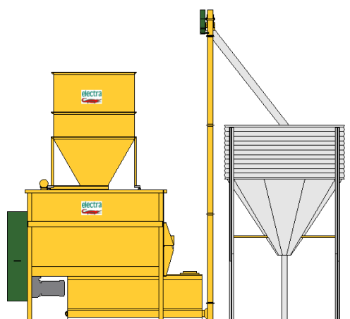
Unité de fabrication 10 t/h
