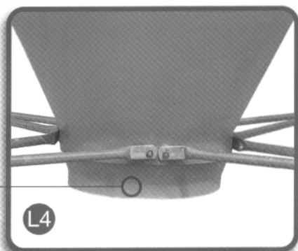
Boitard double trappe sur roulement (pour faciliter le fonctionnement).
