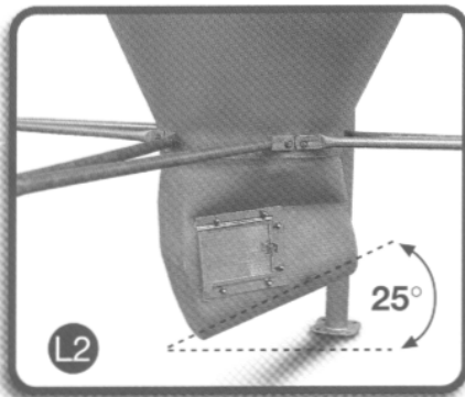
Boitard de reprise par vis 25°.
