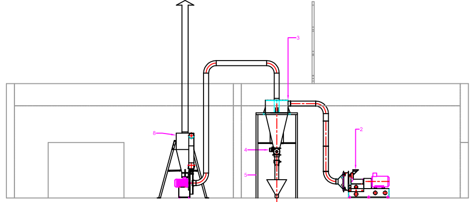
VUE LIGNE DE MICRONISATION DE MANIOC
