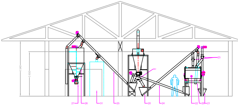
VUE LIGNE DE MELANGE ET CONDITIONNEMENT
