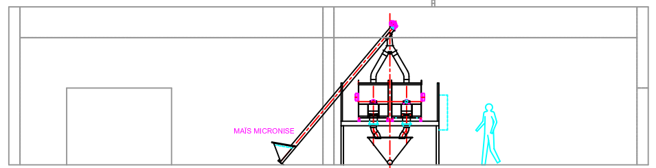
VUE LIGNE DE MELANGE - INCORPORATION MAÏS MICRONISE
