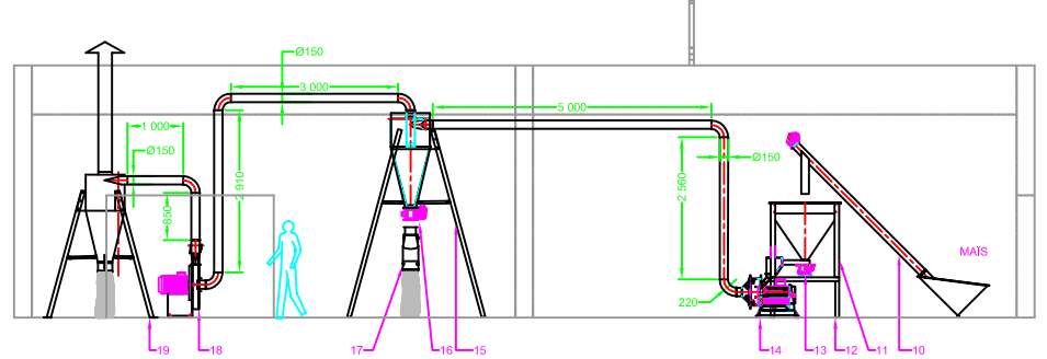
VUE LIGNE DE MICRONISATION EN MAÏS
