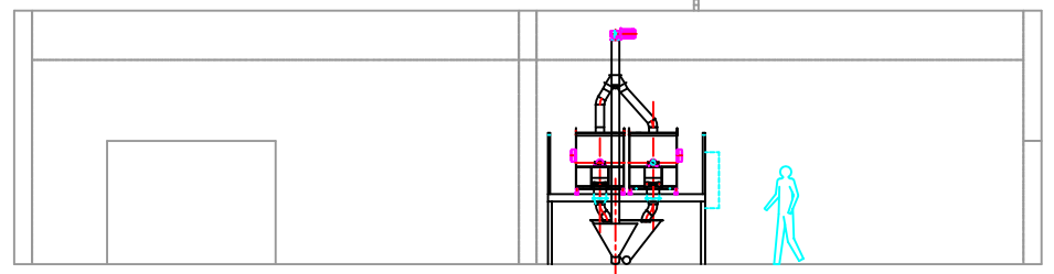
VUE LIGNE DE MELANGE - INCORPORATION MANIOC MICRONISE
