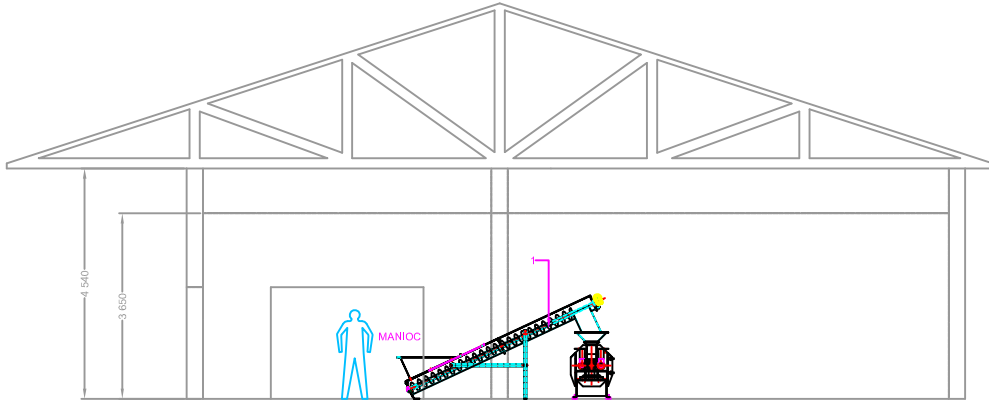
VUE LIGNE DE MICRONISATION DE MANIOC
