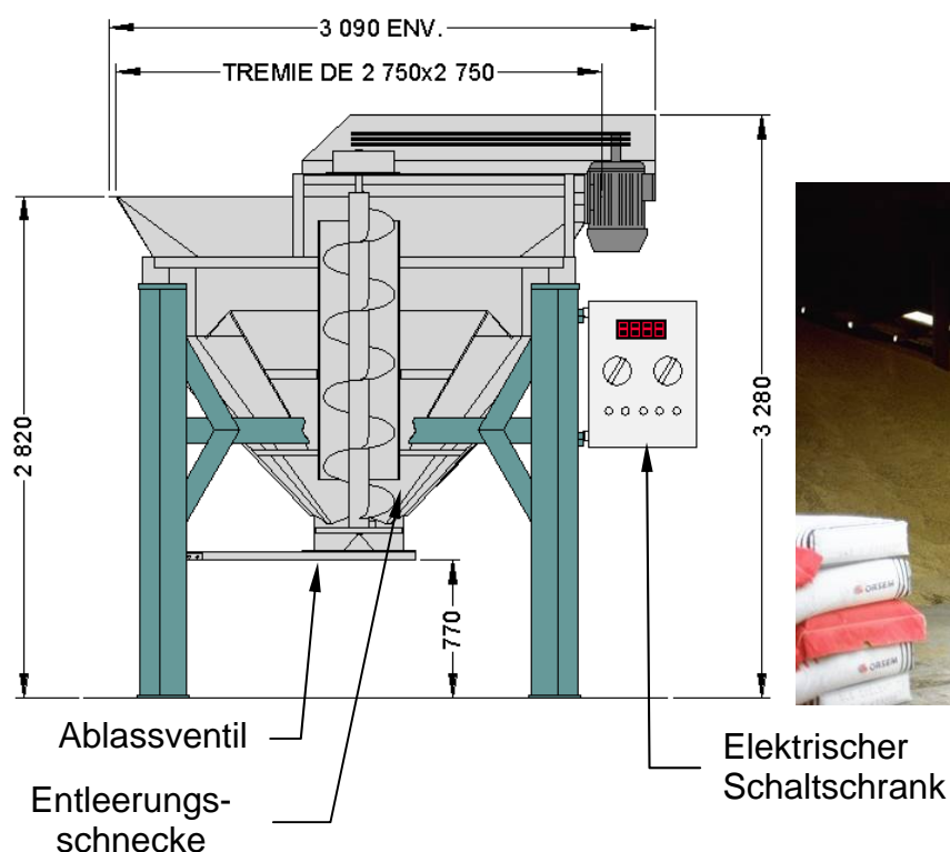
Anwendungsbeispiel einer MV 5000
