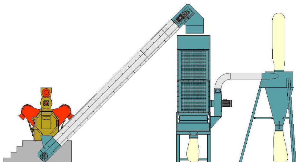
Reprise de granulés en sortie de presse
